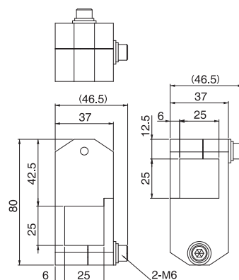
方形滑动支架 • 10-20
