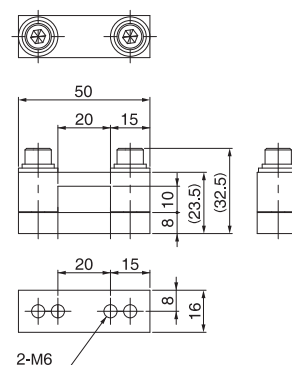
方形滑动支架 • 25-25
