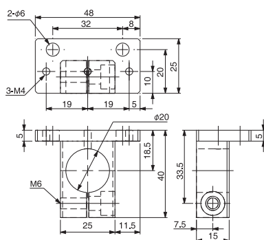
支架·φ20
