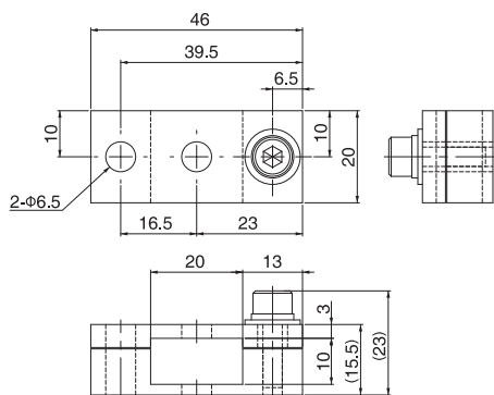
方形滑动支架 • 20-10
