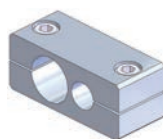
平行连接块· \phi 20 \phi 12
