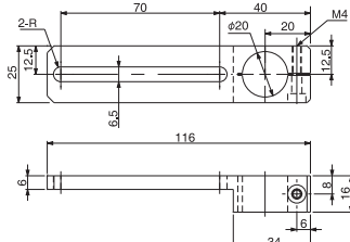
滑移70支架·W· \phi 20 货号No. 131138 规格 N01863-115 ●重量: 48.3g
