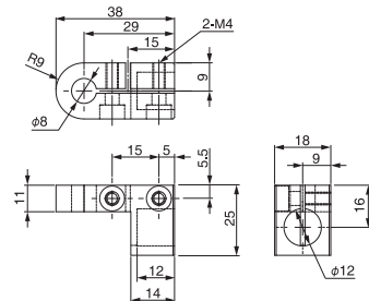
旋转支架· \phi 12 \cdot 12B
