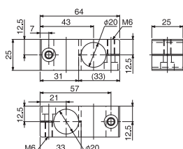
十字连接块 · \phi 20 \phi 20 (后入)
