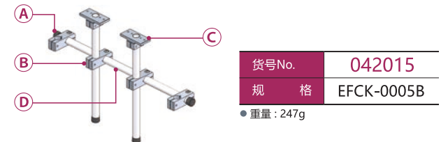
基础框架·钢管系列用
