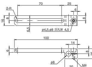
滑移70支架·T·W· \phi 8 货号No. 230053 规格 XL0005-104 ●重量: 25.4g
