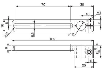
滑移70支架·W· \phi 12 货号No. 131130 规格 N01863-103 ●重量: 24.7g
