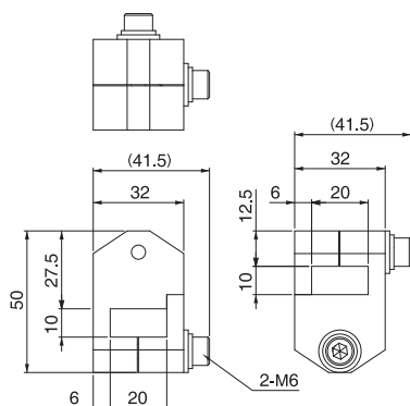
附加支架 • 10-20 • M6
