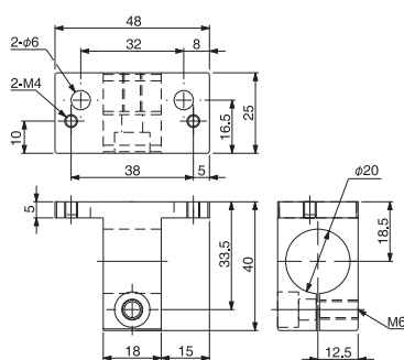
支架·TV·φ20·MCD用
