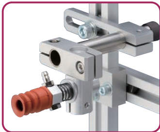
吸着
