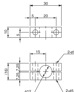
支架·W·φ12
