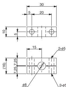
支架·W·φ8
