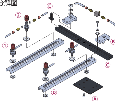
C 标准夹具滑移板
