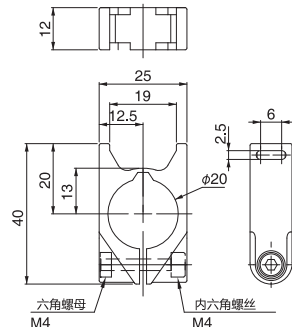
树脂固定φ20 (扎带固定座)
