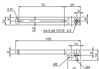
滑移70支架·T· \phi 8 货号No. 230057 规格 XL0005-108 ●重量: 20.0g
