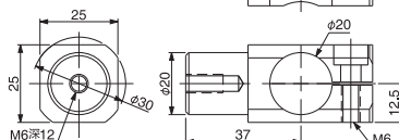
旋转支架· \phi 20 \cdot 20A
