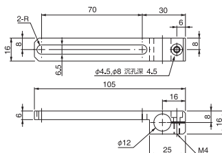
滑移70支架·T· \phi 12 货号No. 230050 规格 XL0005-101 ●重量: 26.2g
