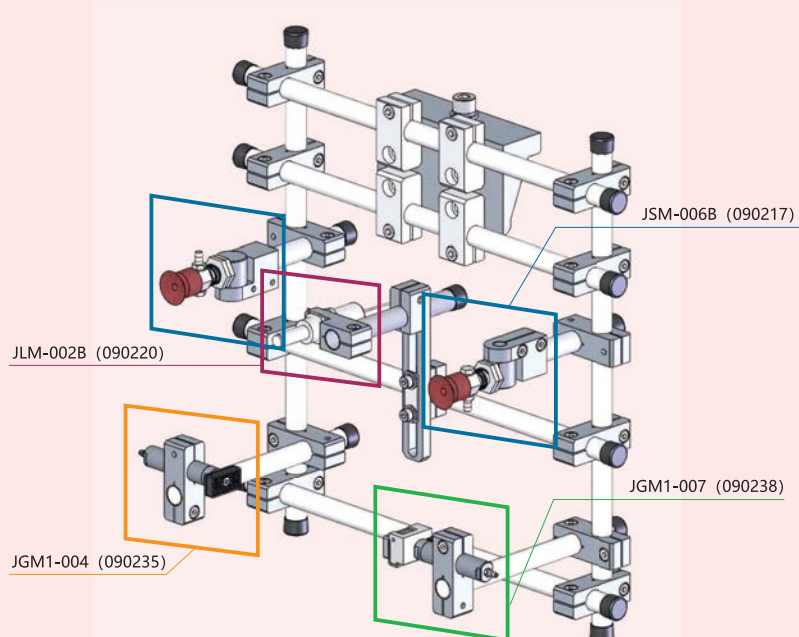
夹持模组
