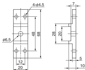
E 标准夹具安装螺丝
