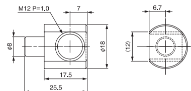
旋转支架· \phi 12 \cdot 8B
