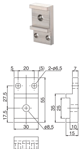
B 标准夹具滑移支架
