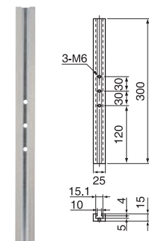
E 标准夹具安装螺丝 H
