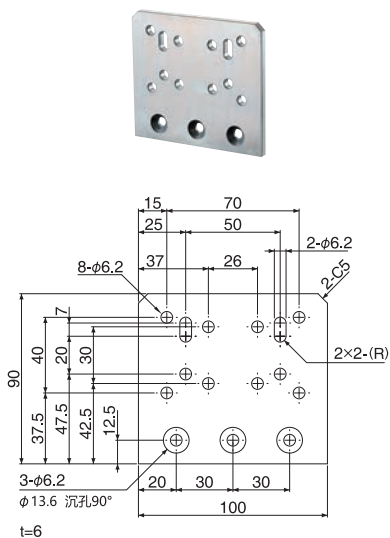
A 标准夹具安装板
