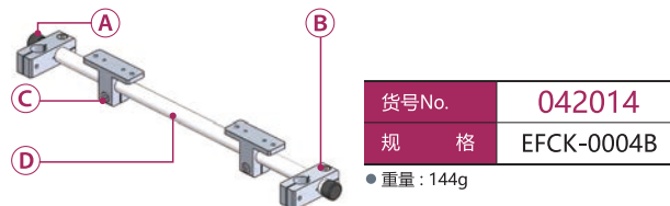
基础框架·钢管系列用
