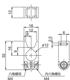
树脂固定φ12 (扎带固定座)
