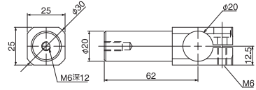
旋转支架· \phi 20 \cdot 20AL
