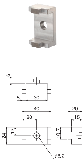
B 标准夹具滑移支架 H
