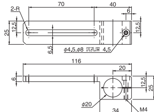
滑移70支架·T· \phi 20 货号No. 230055 规格 XL0005-106 ●重量: 63.7g
