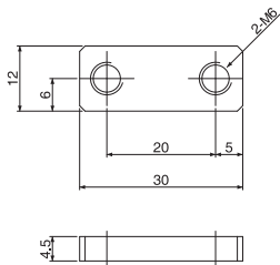
安装板· 滑移支架用 货号No. 023197 规格 CP-076 ●重量: 15.0g
