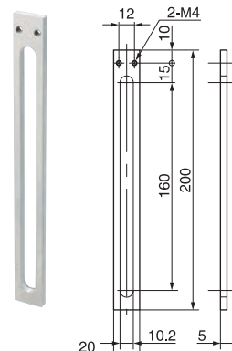
D 标准夹具滑纵杆
